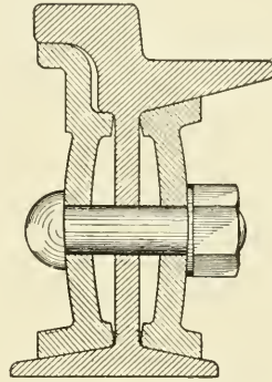
Fig. 224. Girder Rail
